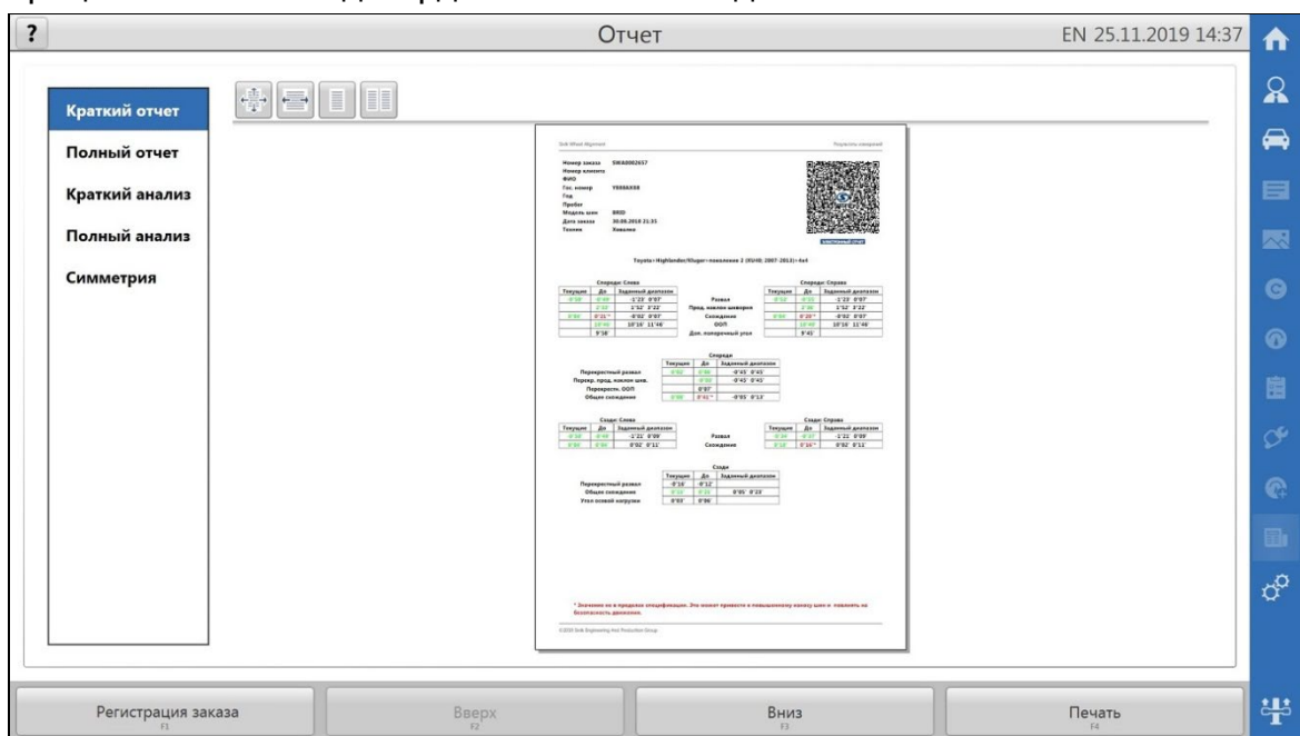
Рисунок 5.29 - Окно отчетов
