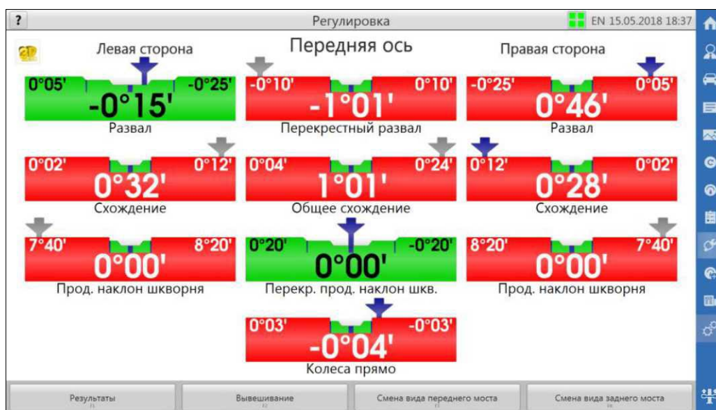
Рисунок 5.26б - Окно регулировки (2D-вид)
